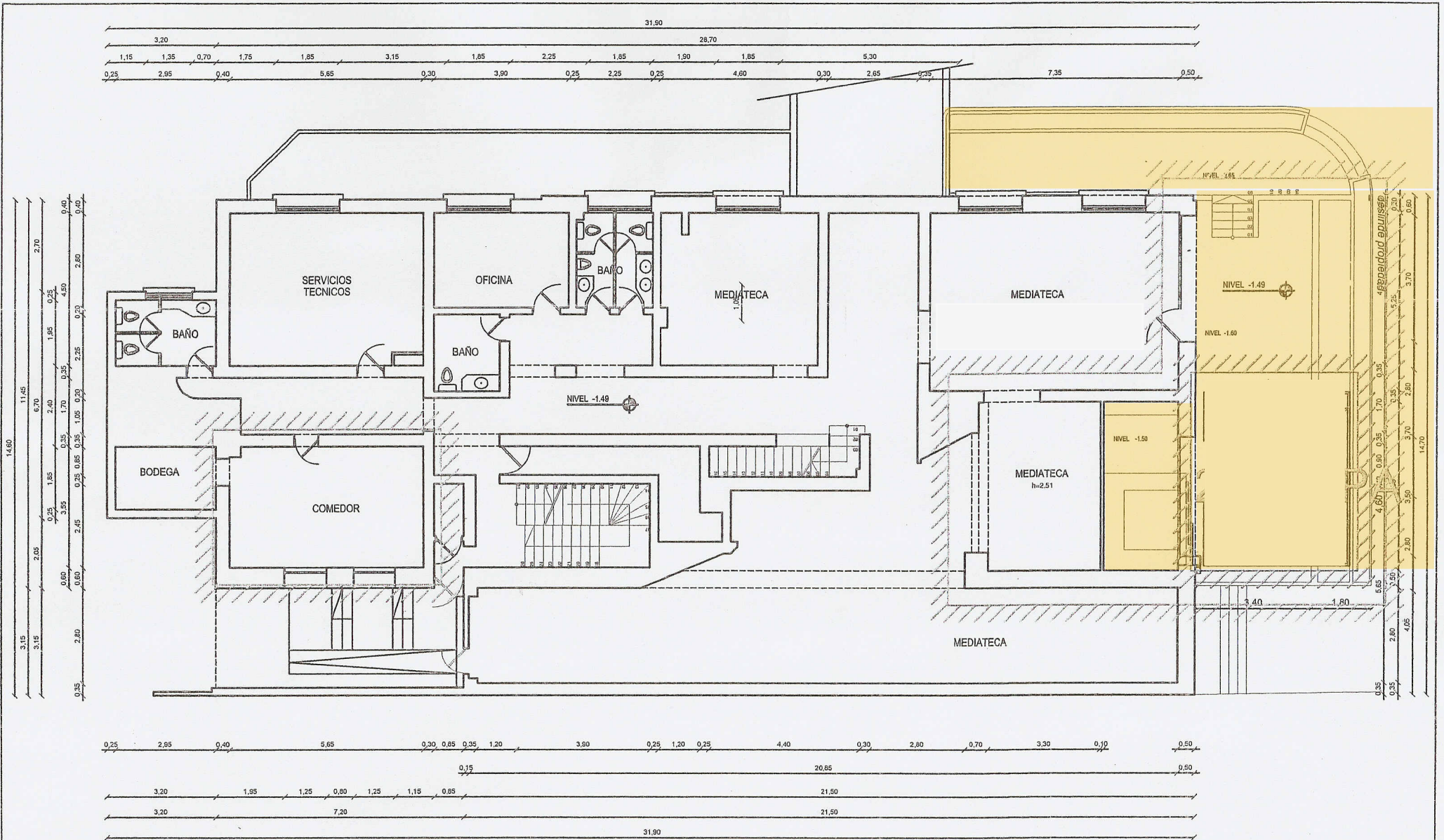
PLANTA NIVEL ZÓCALO REMODELACIÓN ESC. 1:50
